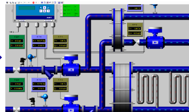
Интерфейс программы диспетчеризации теплового узла ОБЩЕЖИТИЯ № 5
