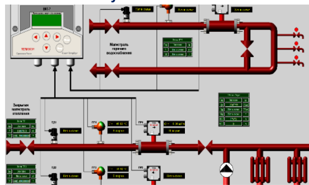
Интерфейс программы диспетчеризации теплового узла ГЛАВНОГО КОРПУСА
